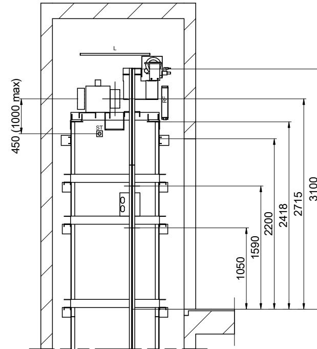
MUR COTE CONTREPOIDS ECHELLE[*]: 1:50
