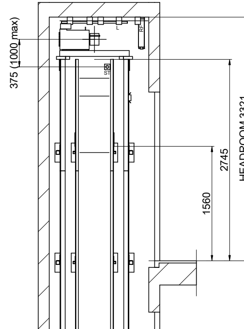
SCALE[*]: 1:50
