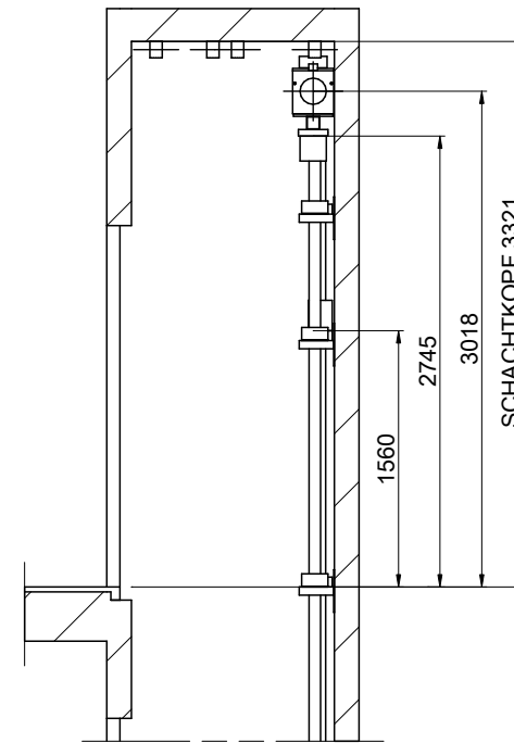
MASSTAB[*]: 1:50
