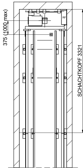
MASSTAB[*]: 1:50
