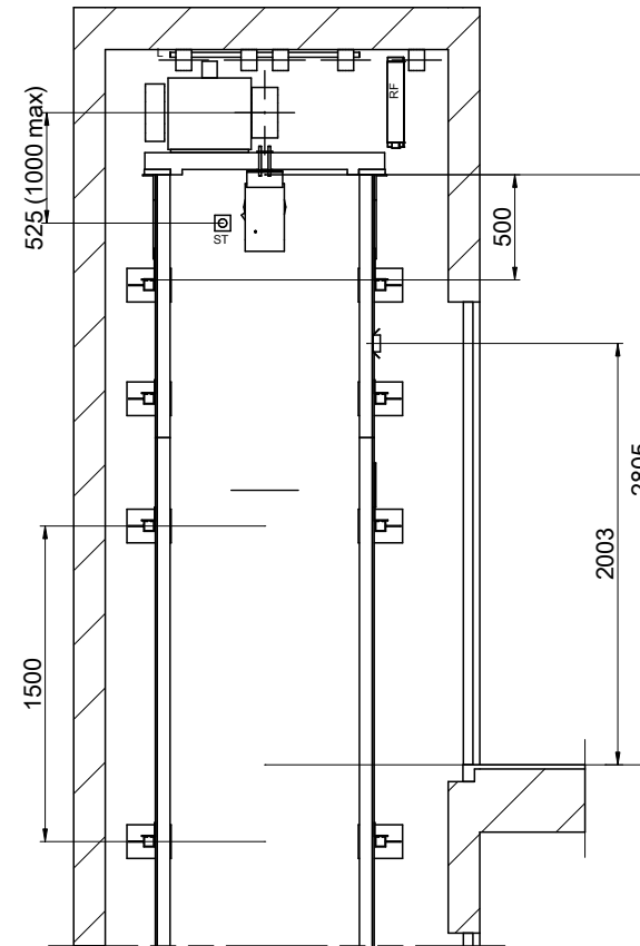
ECHELLE[*]: 1:40
