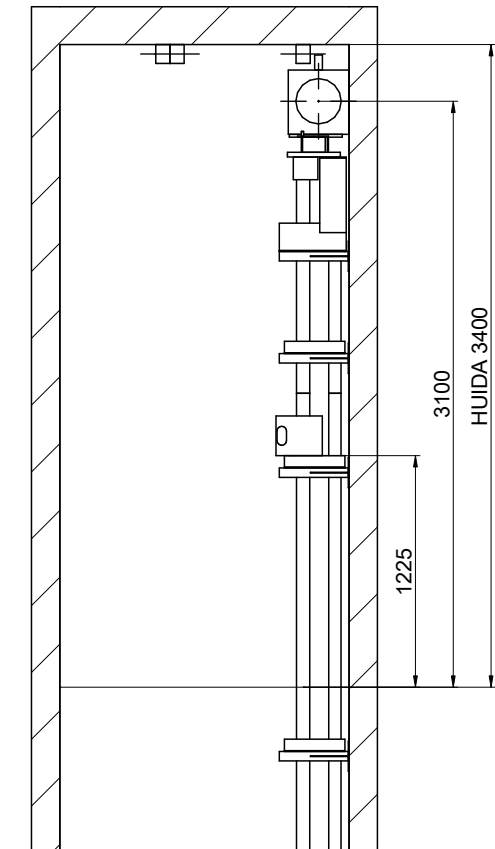
ESCALA[*]: 1:40
