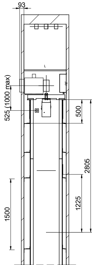
MASSTAB[*]: 1:50
