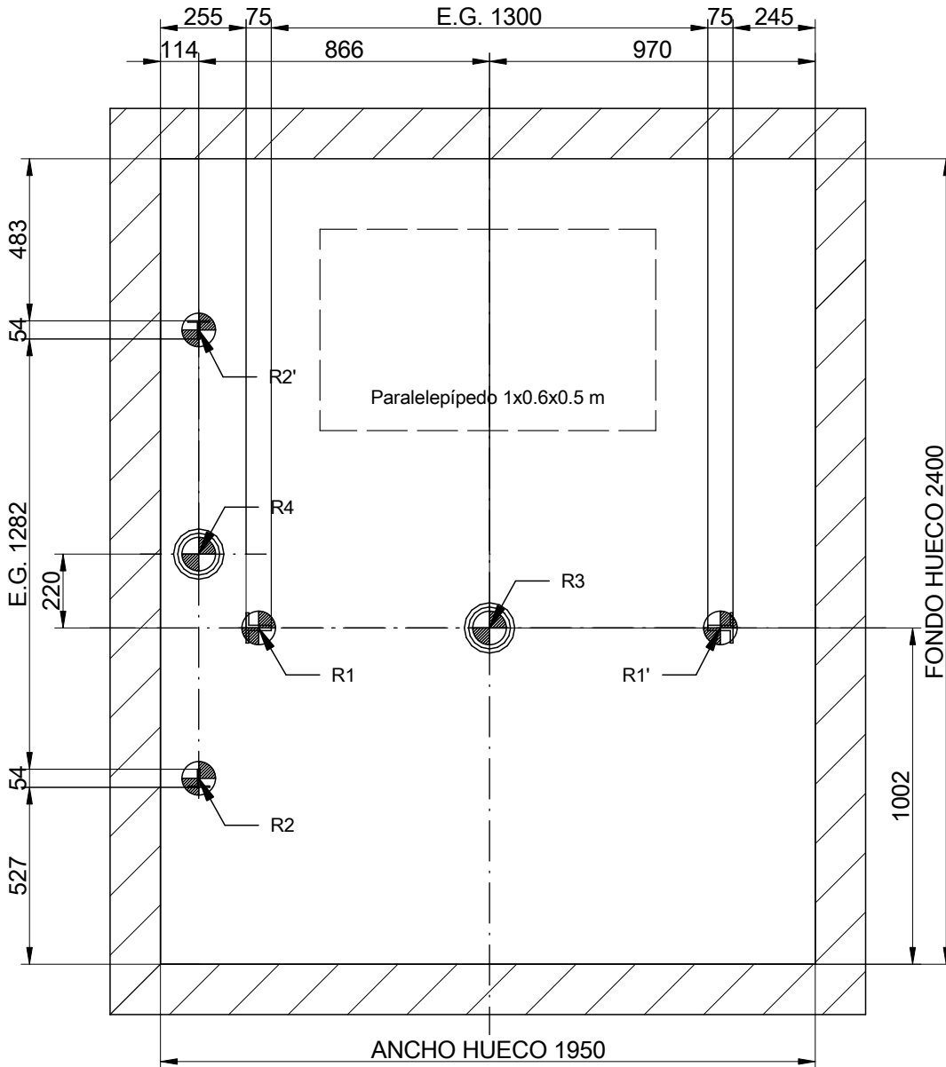
PLANTA DE FOSO ESCALA(¹): 1:20
