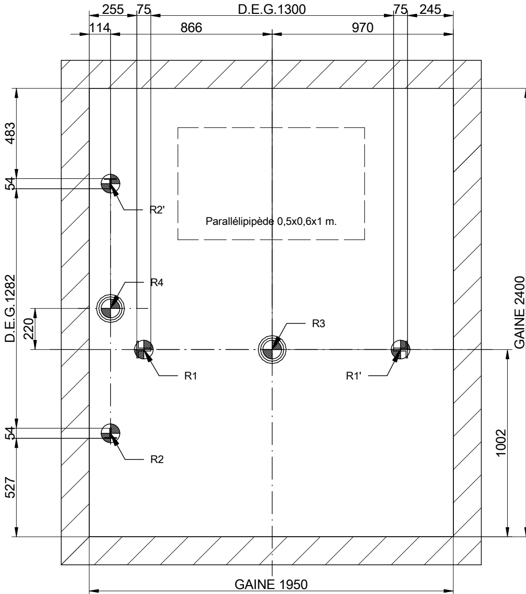
PLAN DE LA CUVETTE ECHELLE(1): 1:20
