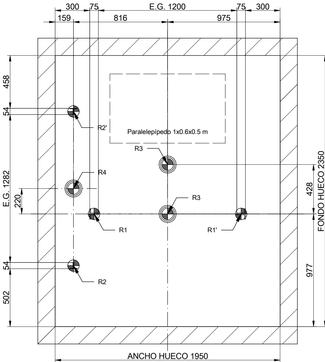
PLANTA DE FOSO ESCALA(1): 1:20
